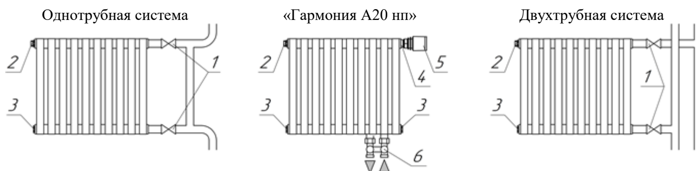
Рис. 2 1. Вентиль. 2. Кран Маевского-воздухоотводчик. 3. Пробка глухая (точка слива). 4. Встроенный термоклав. 5. Термостатический элемент. 6. Запорно-присоединительный клапан нижнего подключения.
